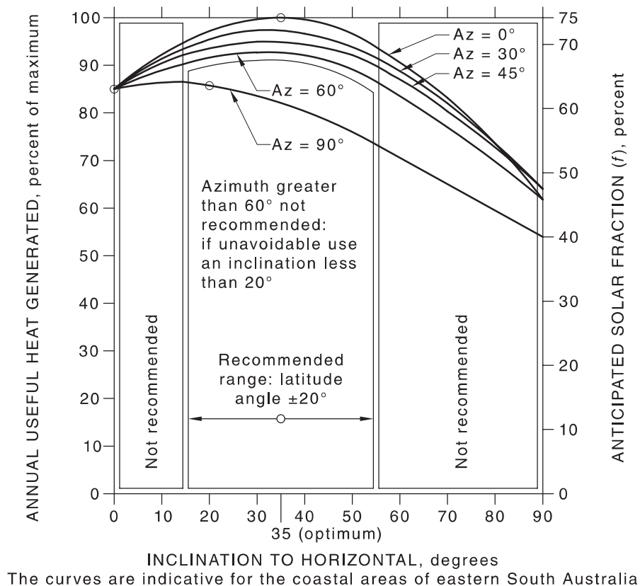
Figure I.1 — Adelaide — Latitude 35°S
