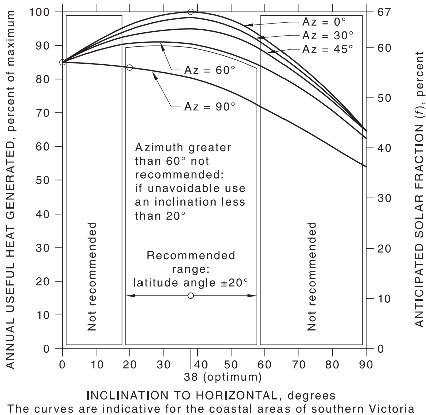
Figure I.7 — Melbourne — Latitude 38°S
