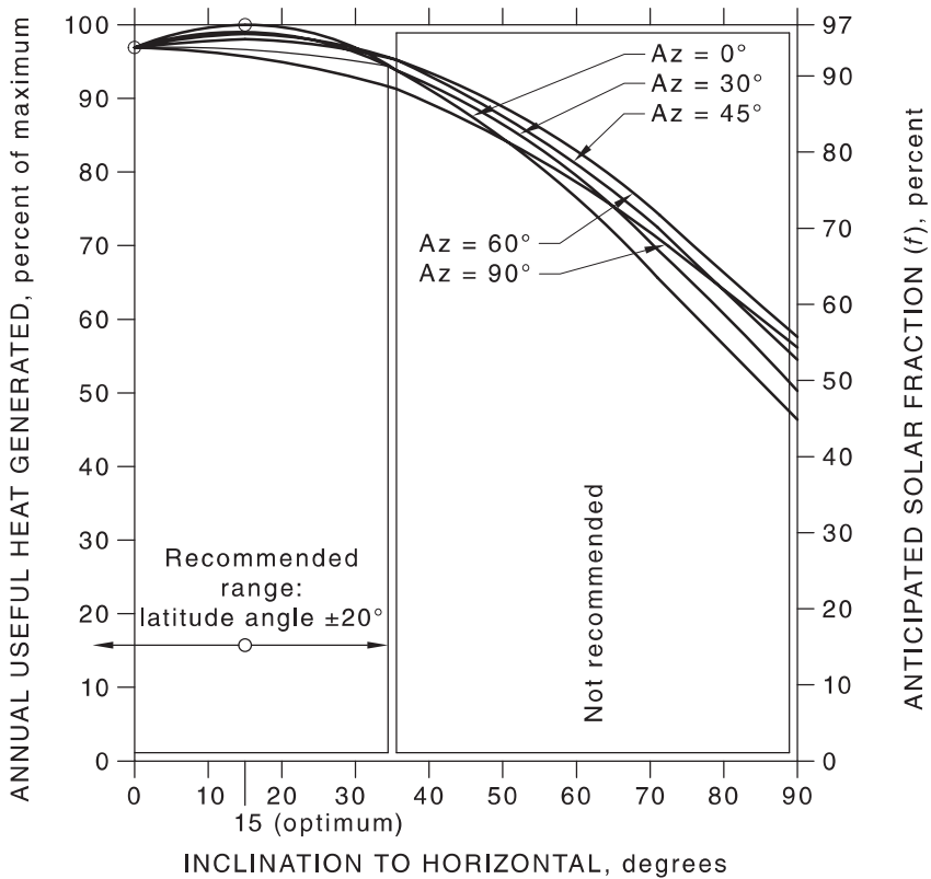
Figure I.4 — Canberra — Latitude 35°S
