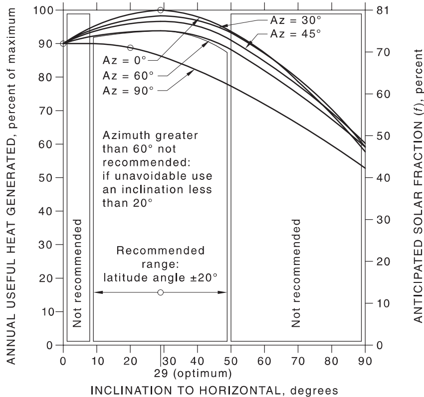
Figure I.2 — Alice Springs — Latitude 24°S
